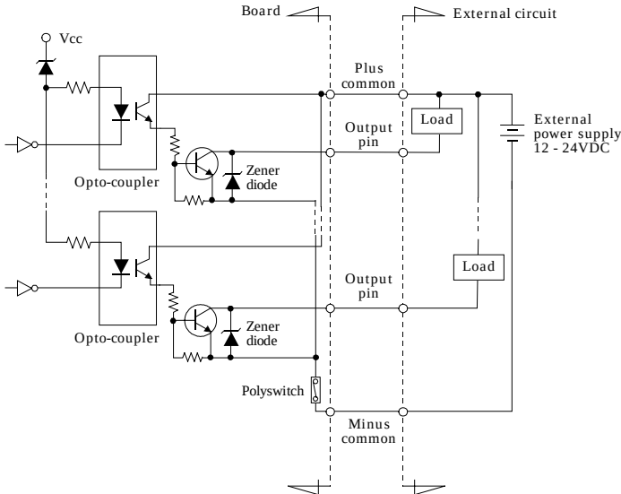
図3.7 出力回路 <DIO-1616L-PE>, <DO-32L-PE>
