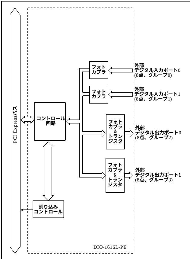
図6.1 回路ブロック図 <DIO-1616L-PE>
