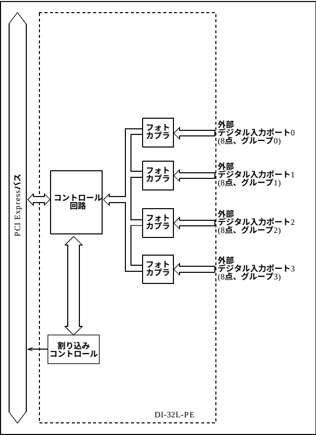
図6.2 回路ブロック図 <DI-32L-PE>
