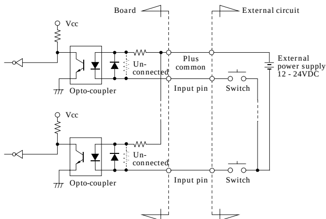
図3.5 入力回路 <DIO-1616L-PE>, <DI-32L-PE>
