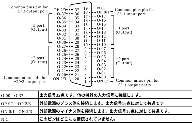
図3.4 インターフェイスコネクタの信号配置 <DO-32L-PE>
