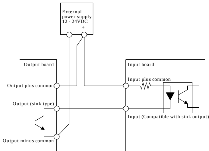
図3.10 シンクタイプ出力とシンク出力対応入力の接続例
