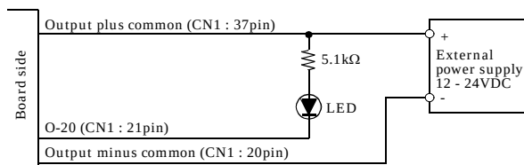
図3.8 出力O-20の使用例 <DIO-1616L-PE>, <DO-32L-PE>
