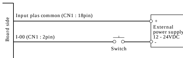
図3.6 入力I-00の使用例 <DIO-1616L-PE>, <DI-32L-PE>
