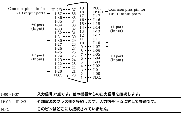
図3.3 インターフェイスコネクタの信号配置 <DI-32L-PE>
