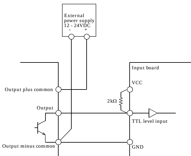
図3.9 出力とTTLレベル入力の接続例 <DIO-1616L-PE>, <DO-32L-PE>
