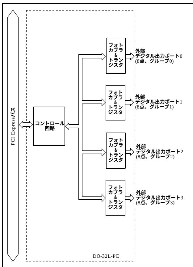
図6.3 回路ブロック図 &lt;DO-32L-PE&gt;
