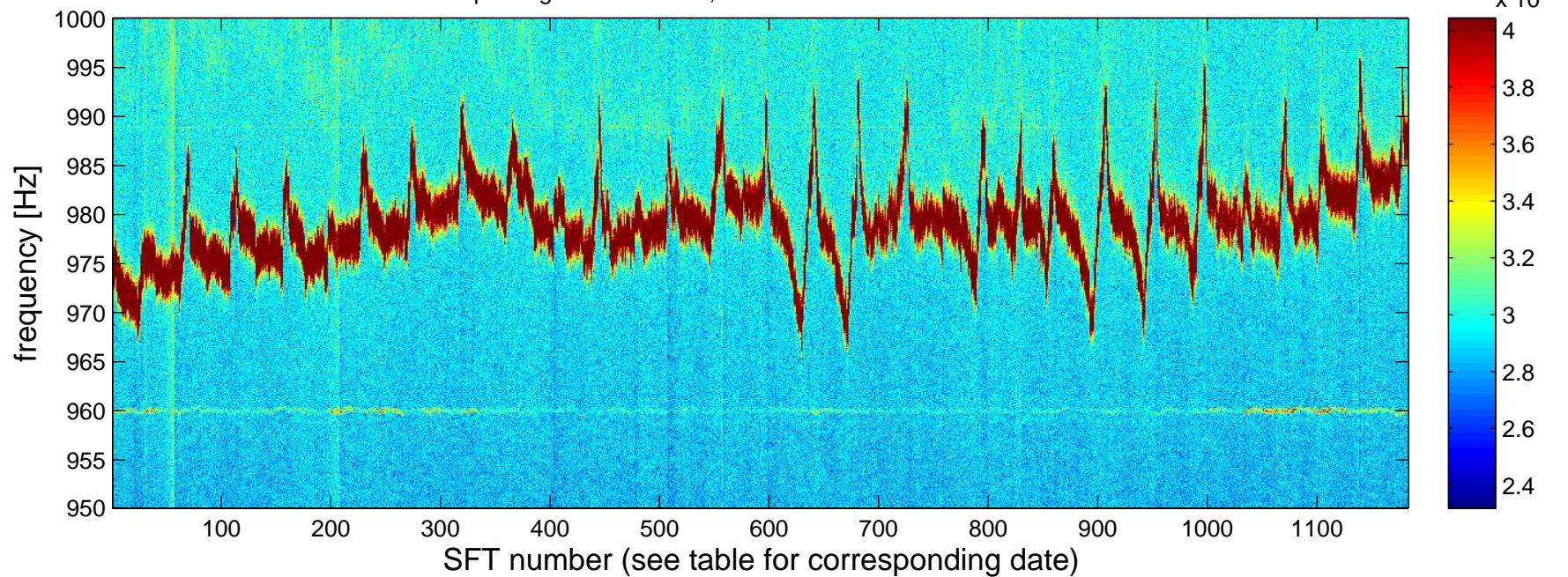
Spectrogram for H1:hoft; GPS 841104014 – 843696014 s.
